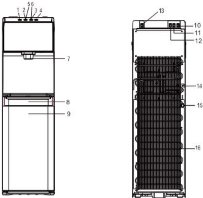
Рисунок 1. Схема аппарата 450ASM
